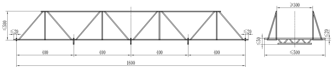
图 18 模型尺寸要求
