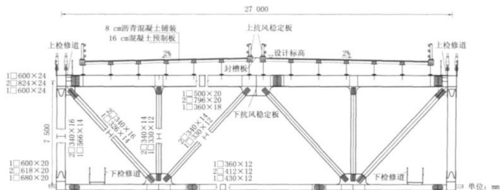
图 2 矮寨特大桥梁体桁架示意图
