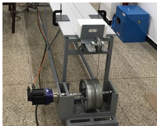
图 15 移动加载驱动装置
